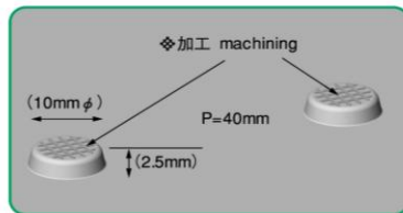
図1:すべらんなーⅠ 断面形状(凸部拡大)
