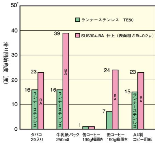
図1 ランナーステンレスの滑り開始角度
