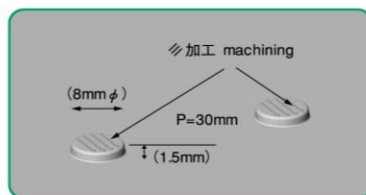
図2:すべらんなーⅡ 断面形状(凸部拡大)
