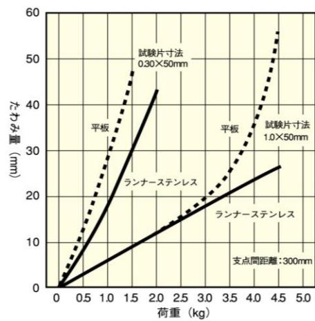
図2 ランナーステンレスの剛性の向上
